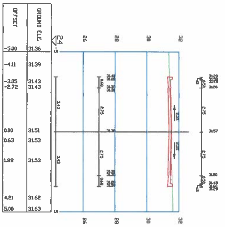
SECTION 0+050 St. 50 Rogozului
