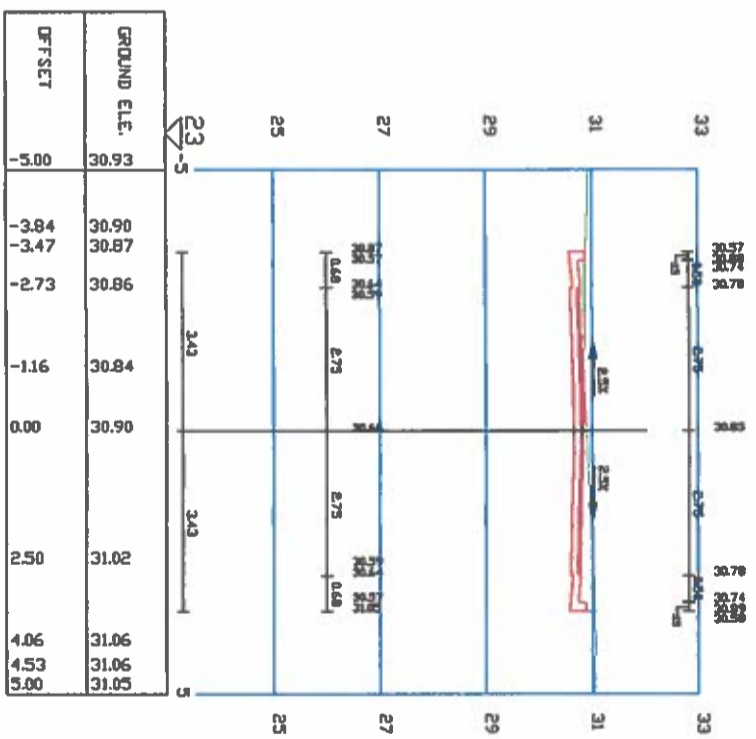
SECTION 0+125 St. 125 Rogozului
